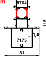
70-7012-11825 1.880 kg/m
