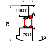
70-1734-1735 1.481 kg/m
