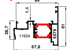
64-1728-1729 1.407 kg/m
