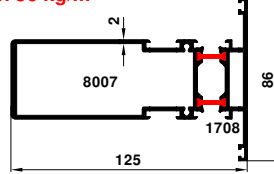
64-5547-1953 1.649 kg/m
