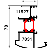
55-1734-1735 1.465 kg/m
