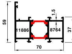
70-7038-7005 1.737 kg/m
