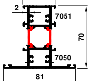
70-7051-7050 2.083 kg/m
