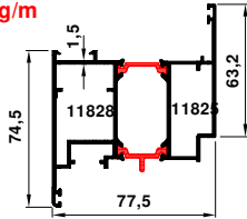
70-7028-7029 2.542 kg/m
