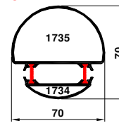
55-1734-1735 1.465 kg/m
