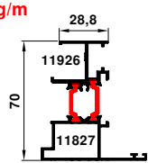
70-11926-11827 1.280 kg/m
