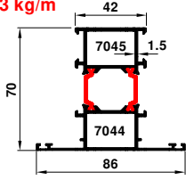
70-7010-11824 1.570 kg/m
