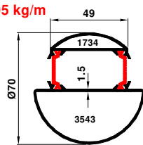
64-1734-3543 1.405 kg/m
