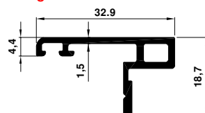
7180 0.244 kg/m
