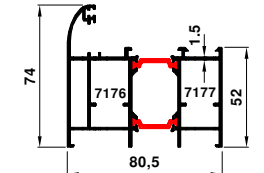
70-7016-7009 1.432 kg/m
