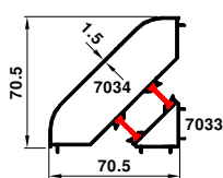
70-11926-11827 1.280 kg/m
