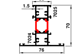
70-8764-8763 1.680 kg/m
