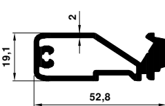
7060 1.007 kg/m
