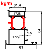
64-1728-1729 1.407 kg/m
