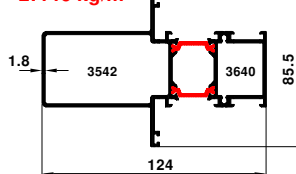
64-1734-3543 1.405 kg/m
