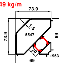
64-5547-1953 1.649 kg/m
