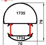
70-1734-1735 1.481 kg/m
