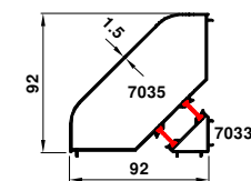
70-11927-11827 1.290 kg/m
