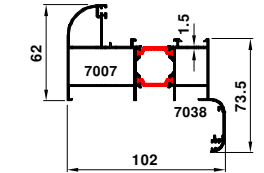
70-7176-7177 2.017 kg/m
