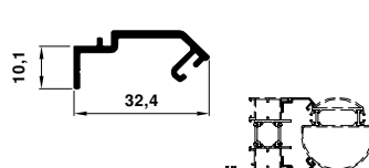
7180 0.244 kg/m
