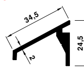
1011 0.402 kg/m
