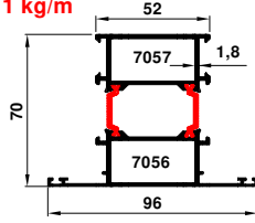
70-7017-11824 1.537 kg/m
