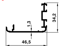
2703 0.403 kg/m
