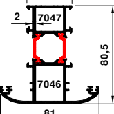
70-7047-7046 2.129 kg/m
