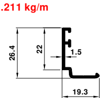
1912 0.211 kg/m
